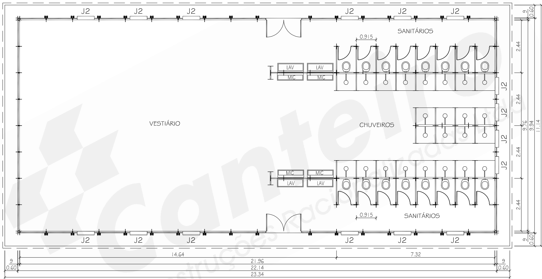
PLANTA
