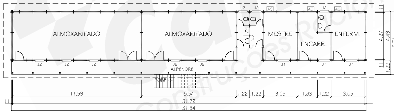
PLANTA - PAVIMENTO INFERIOR
