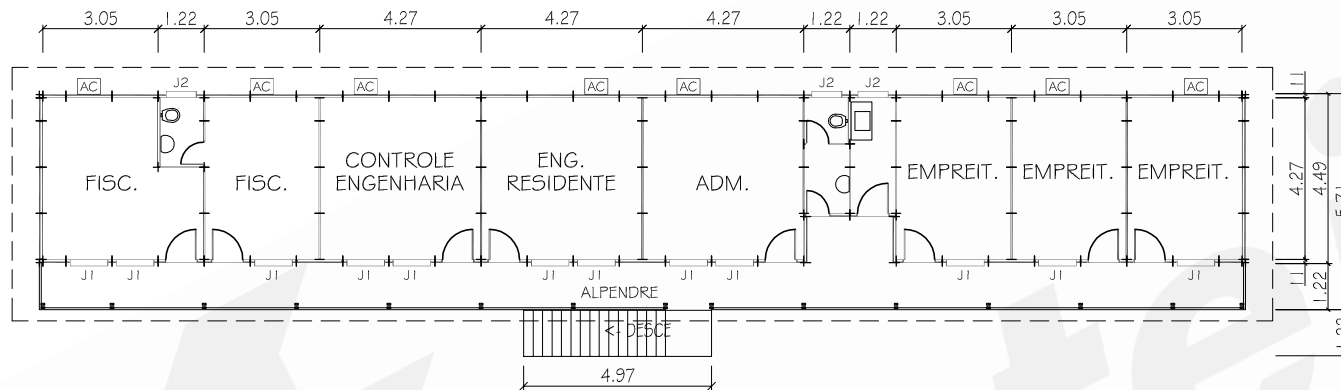
PLANTA - PAVIMENTO SUPERIOR
